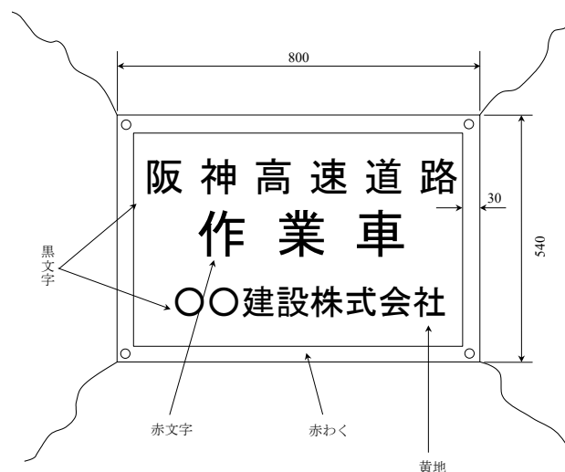
図-3.9.1 工事用車両の明示幕（参考）
