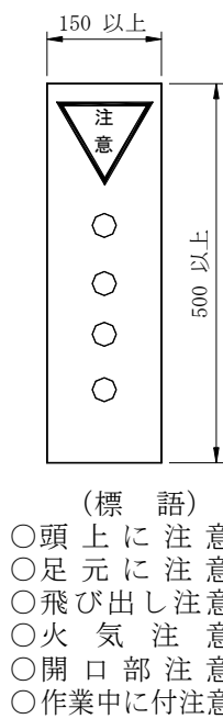
図-3.3.7 注意標識
