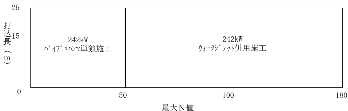
図③-2-3-2 油圧式バイブロハンマ機種の選定範囲
