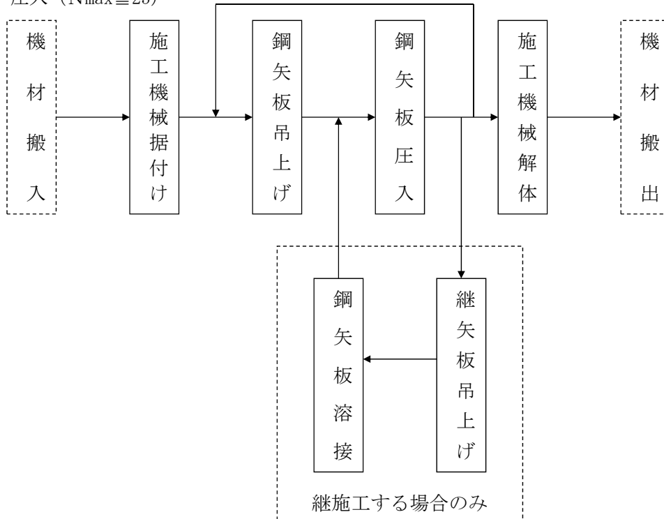
図③-4-2-1 施工フロー（圧入 ( N_{\max} \leq 25 )）
