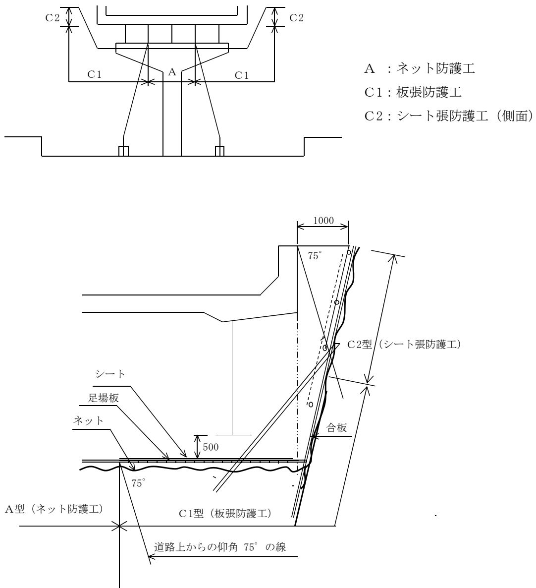
参考図（落下防護工）
