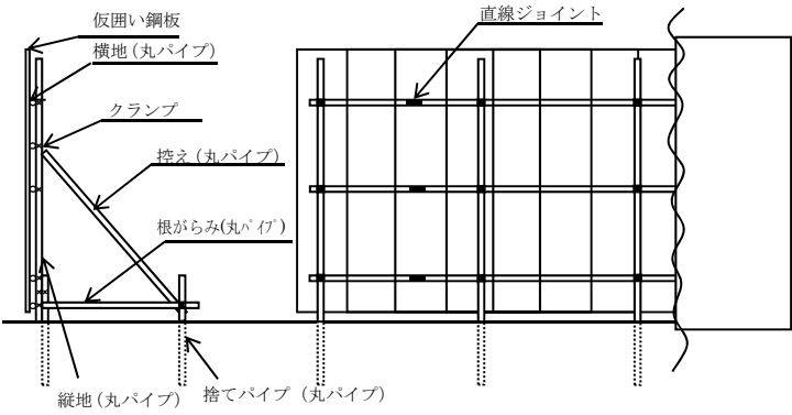
仮囲い概念図（参考）
