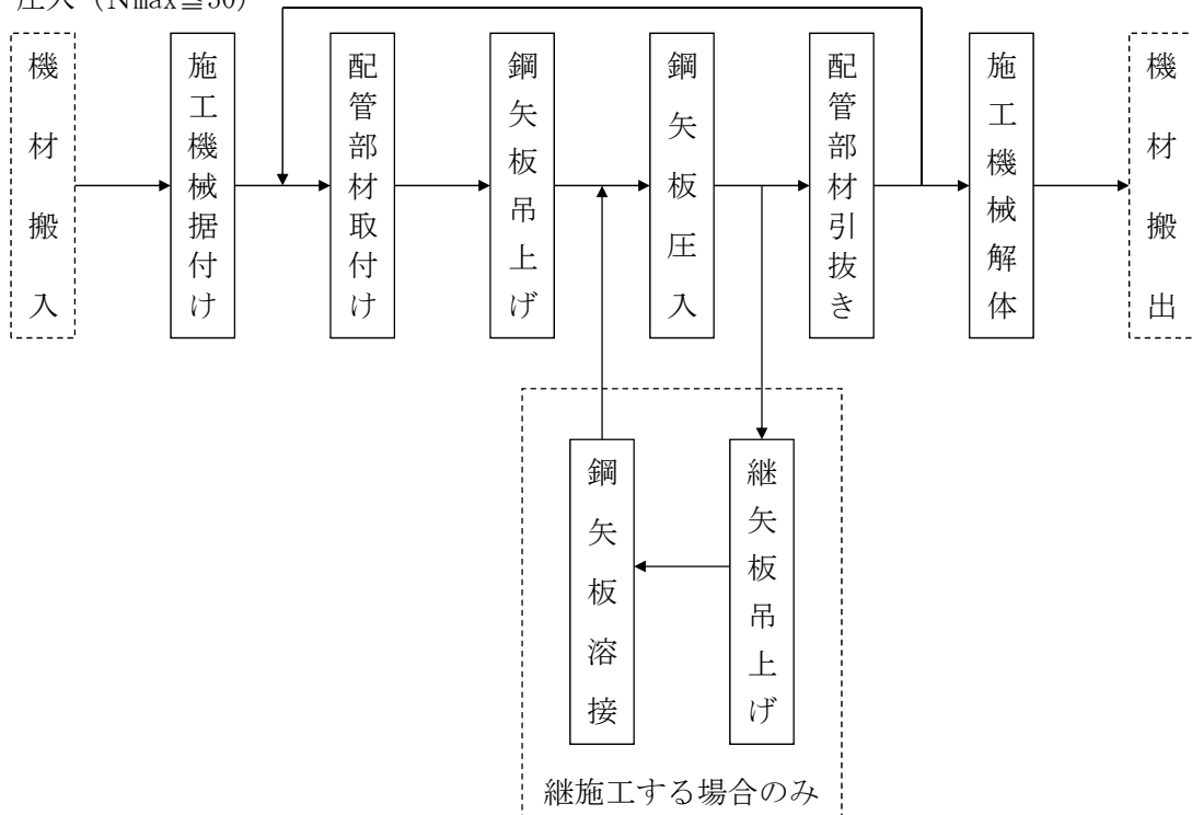
図③-4-2-2 施工フロー（圧入 ( N_{\max} \leq 50 )）
