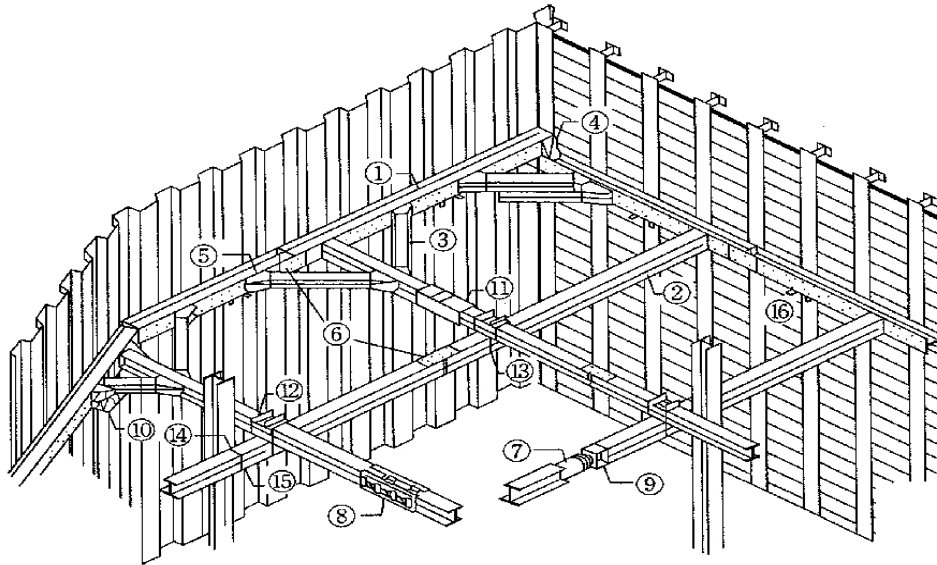
土留標準図
