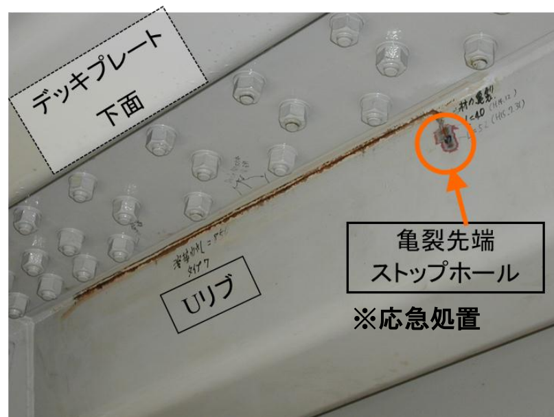
鋼床版のデッキプレートとUリブ 溶接部のき裂
