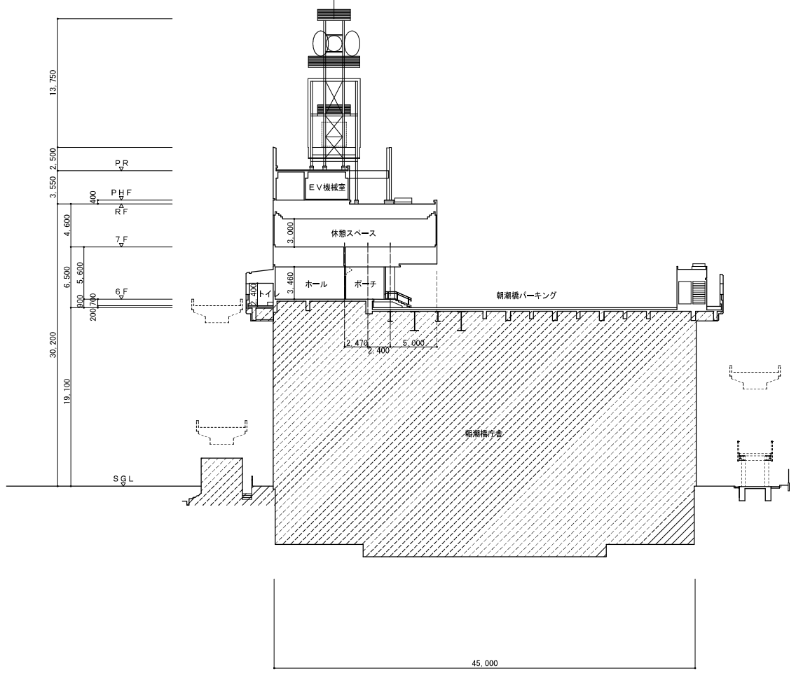
断面図 1/200
