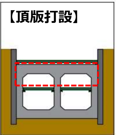
(7) 切梁を外し、 頂版を打設する。
