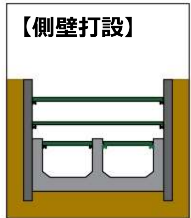
(6) 切梁を外し、 側壁を打設する。
