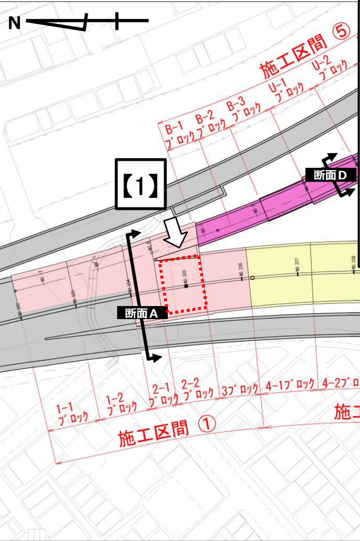
【1】施工区間① 2-2ブロック掘削状況
