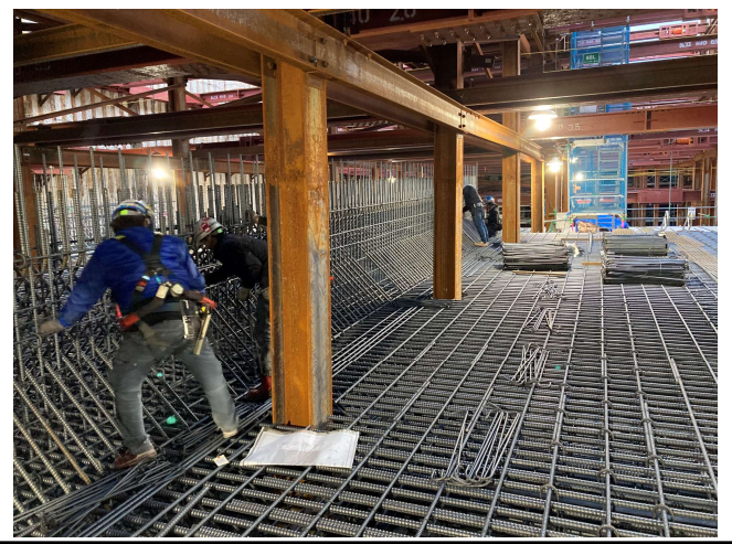
【2】施工区間④ 9-2ブロック 底版鉄筋組立状況
