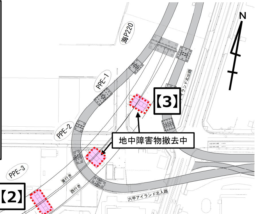
【3】高速道路の橋脚(PPE-1)基礎工事において、地中障害物の撤去中。
