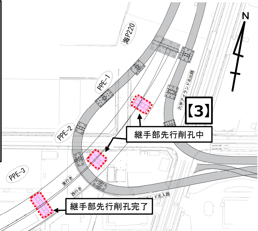
【3】橋脚(PPE-1)基礎工事中において、鋼管矢板継手部の先行削孔状況。
