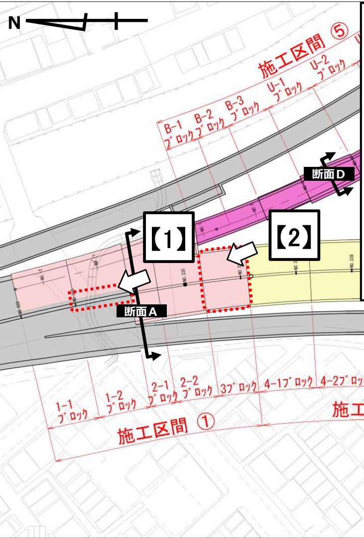
【1】施工区間① 1-2ブロック 既設函体と接続するため、一部函体の研(はつ)り工実施状況
