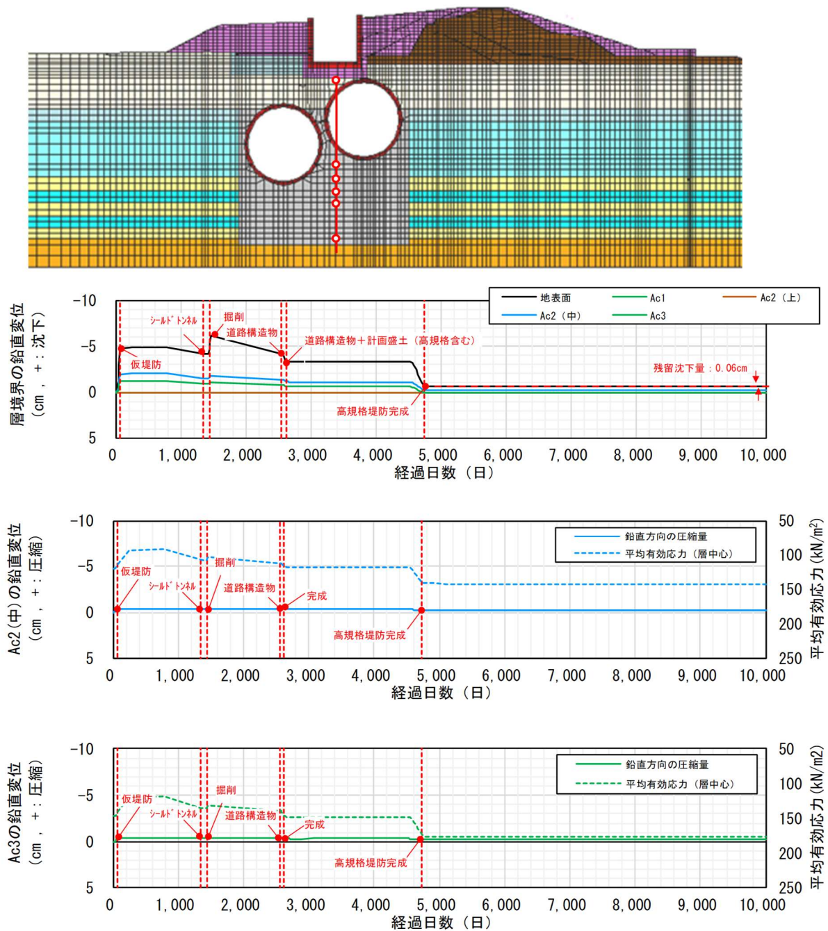
図 5.2.2-7 道路ボックス中央部における地盤変状挙動，応力状態の経時変化
