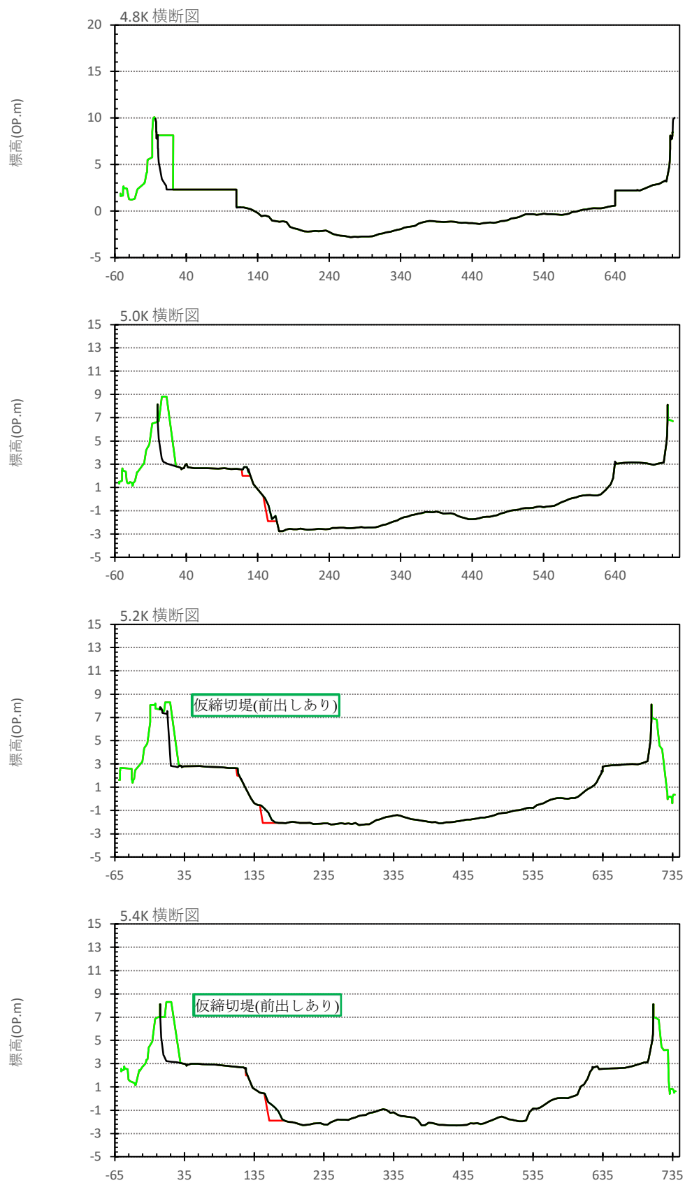
図 6.3.2-3(3) 不等流計算横断(3.8k~9.2k)
