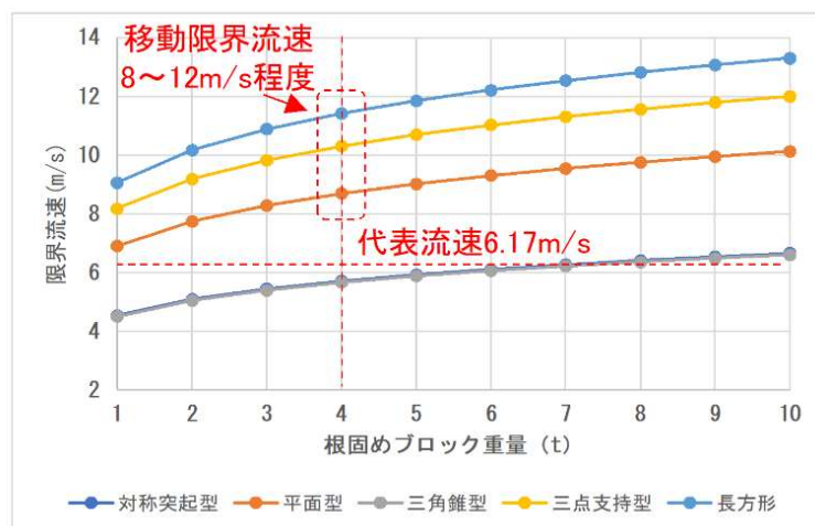
図 6.3.1-5 限界流速と根固めブロック重量の関係
