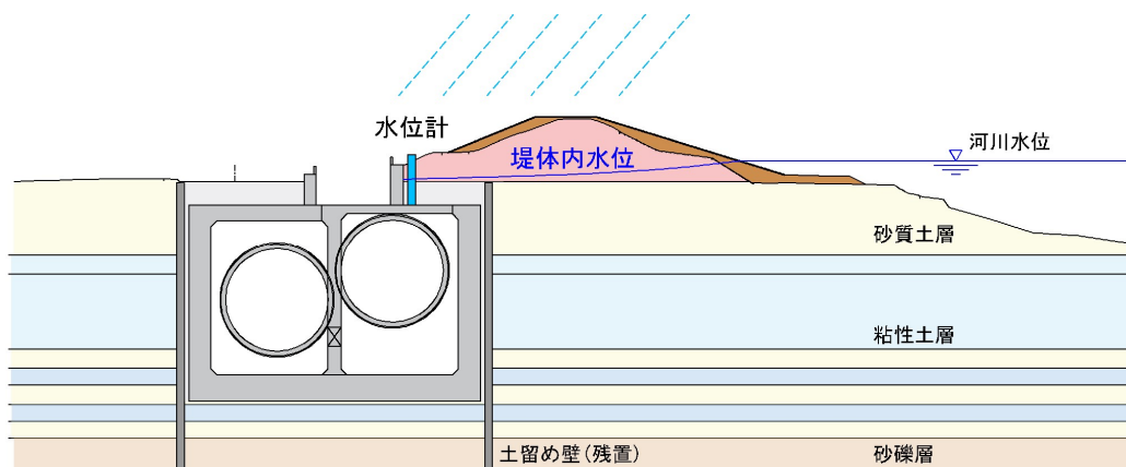
図 7.3.3-1 管理値に関わる堤体内水位の計測位置
