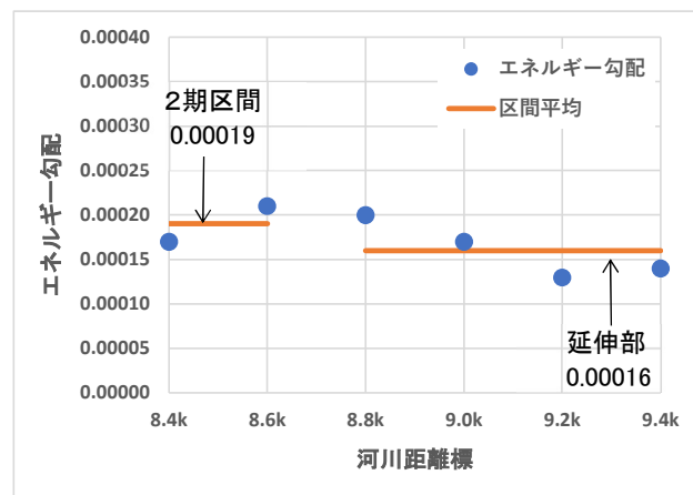
図 6.3.1-1 エネルギー勾配の設定
