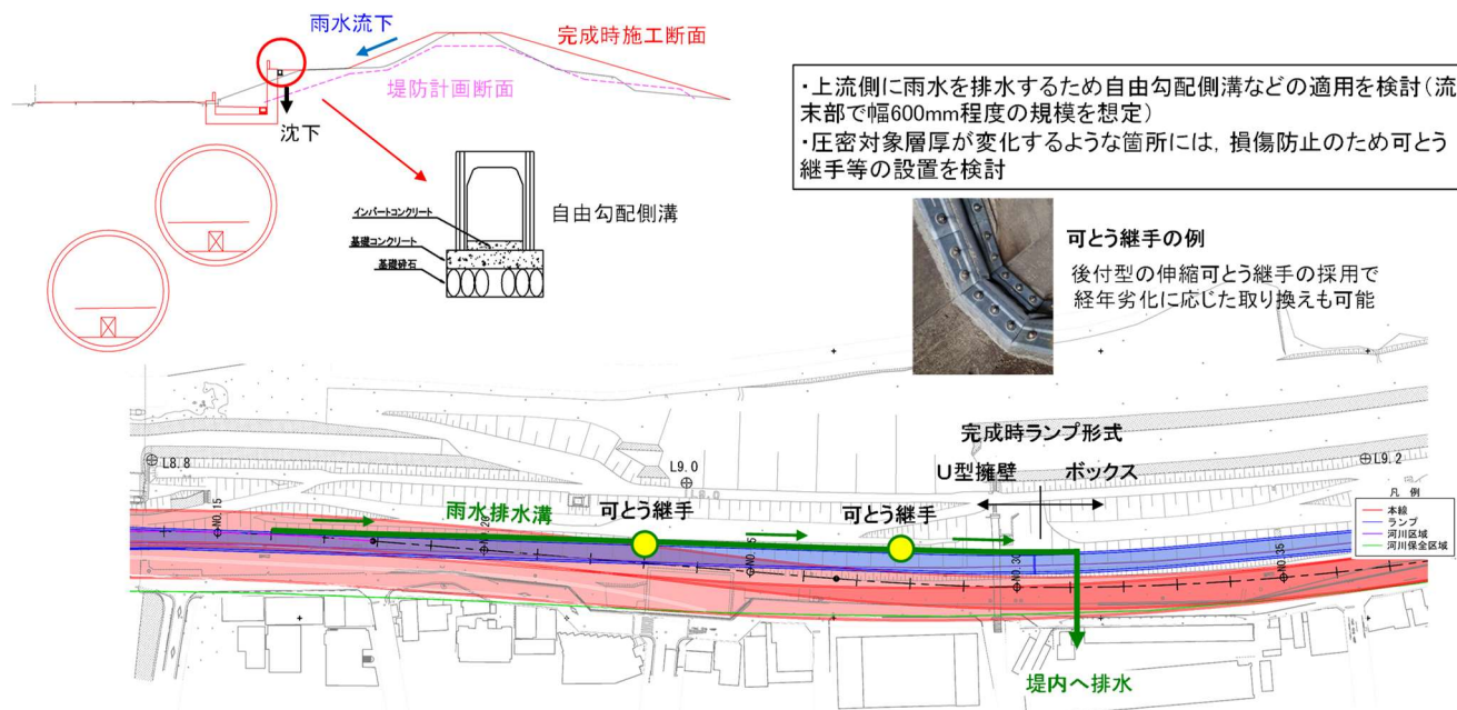
図 7.3.5-2 堤防表面の雨水排水対策例
