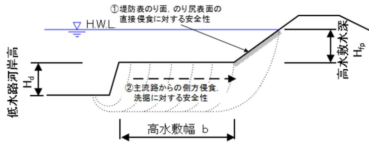
図 6.3.1-6 護岸がない場合の堤防崩壊メカニズム
