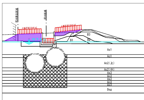
図 5.2.2-4 解析ステップ (3)
