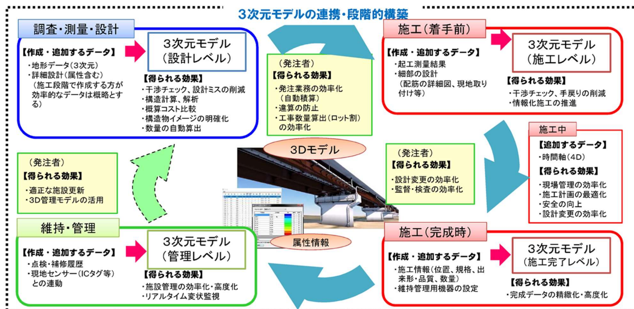
図 7.3.6-1 維持管理を含めた 3 次元モデルの連携・段階的構築の例
