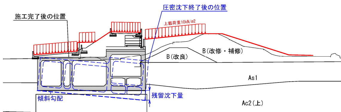
図 5.2.2-1 圧密沈下に伴う堤防高の確保の照査方法
