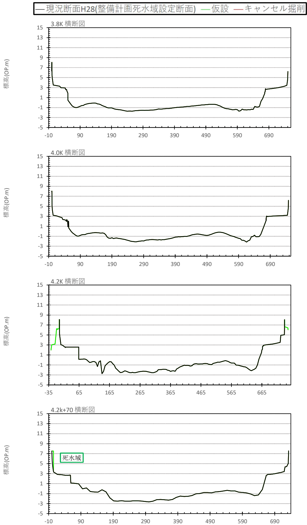
図 6.3.2-3(1) 不等流計算横断(3.8k~9.2k)
