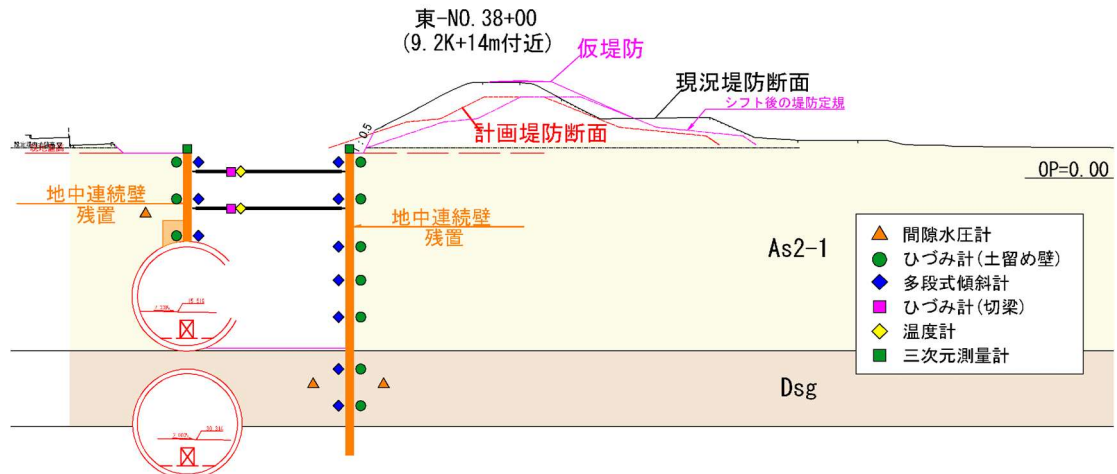
図 6.4.1-1 土留め壁に対する計測の例
