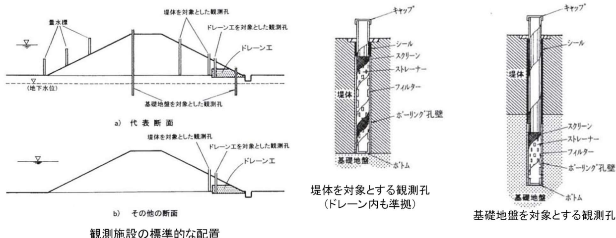
図 7.3.5-6 水位観測施設の標準的な配置と水位観測孔の標準的な構造
