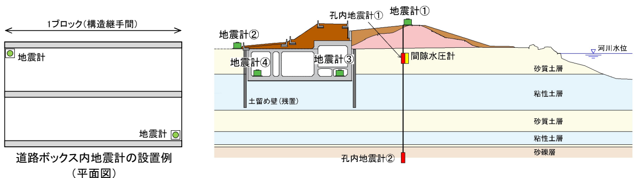
図 7.2.3-1 地震計と間隙水圧計の設置例（開削ボックス区間）
