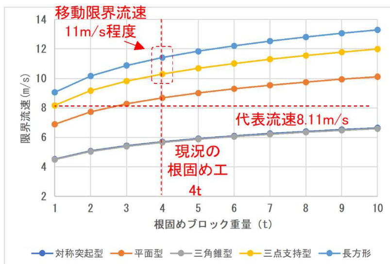
図 5.4.2-10 限界流速と根固めブロック重量の関係
