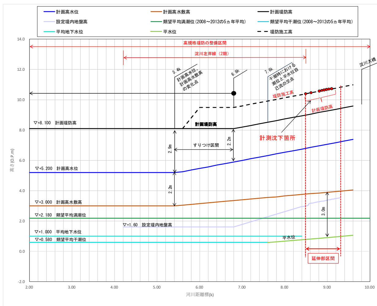
図 7.3.3-2 地表面沈下の管理値の設定例
