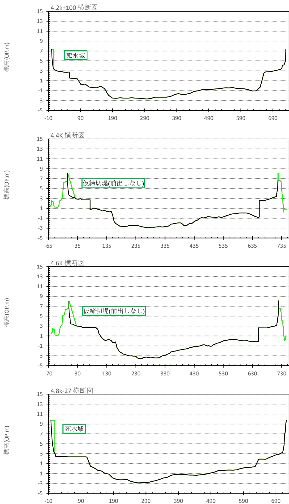
図 6.3.2-3 (2) 不等流計算横断(3.8k~9.2k)
