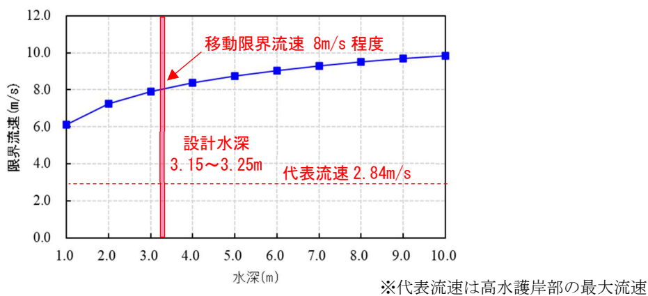
図 6.3.1-4 水深と限界流速の関係（高水護岸における覆土ブロック）
