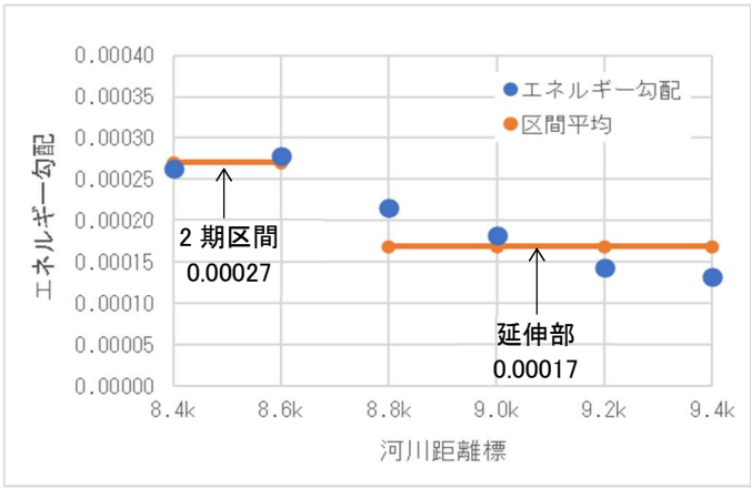
図 5.4.2-7 エネルギー勾配の設定
