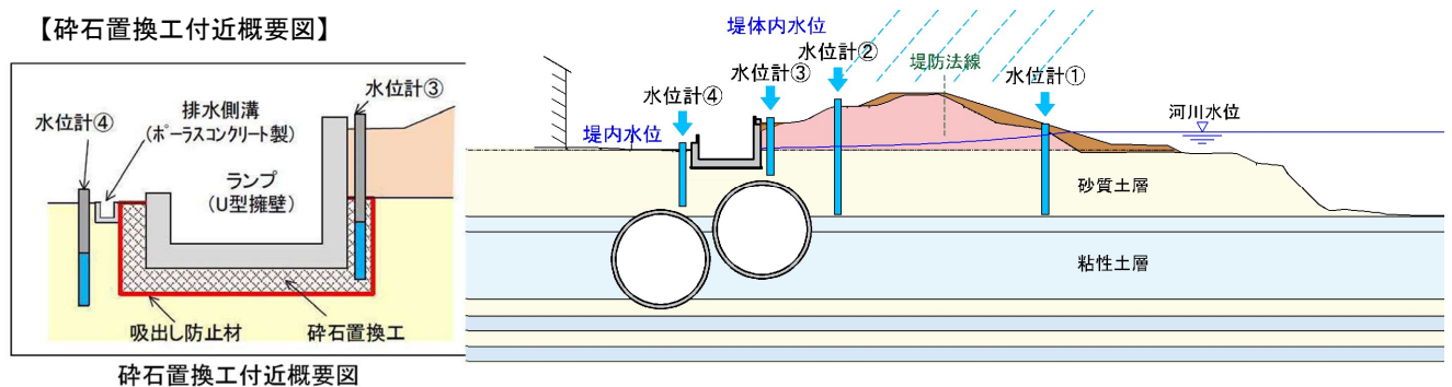
図 7.2.1-2 解析の妥当性検証に用いる水位計測箇所（シールドトンネル区間）
