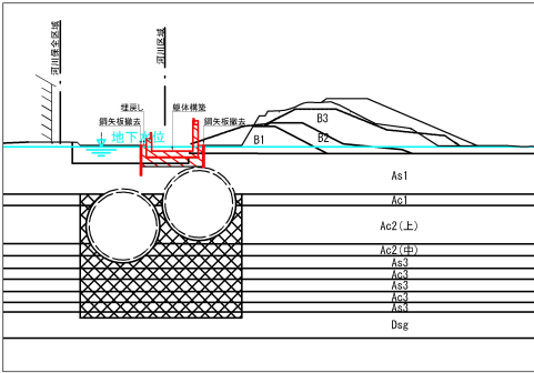
図 5. 2. 2-3 解析ステップ (2)
