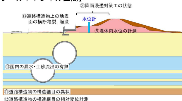
図 7.3.4-2 浸透・パイピングに関連するモニタリング項目
