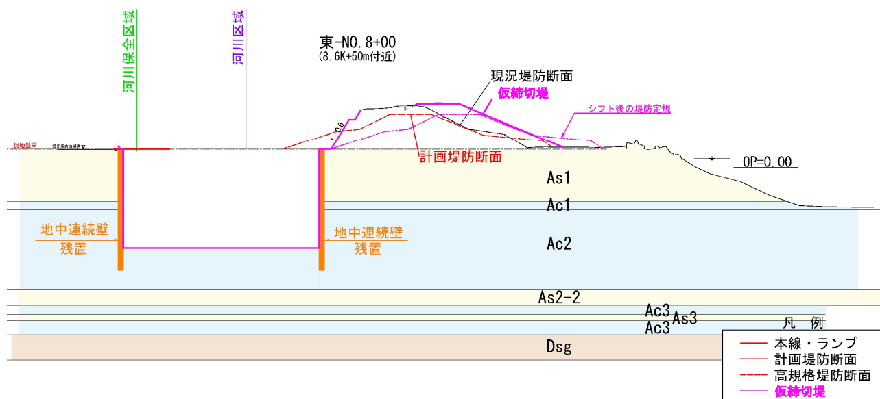
仮締切堤横断面
