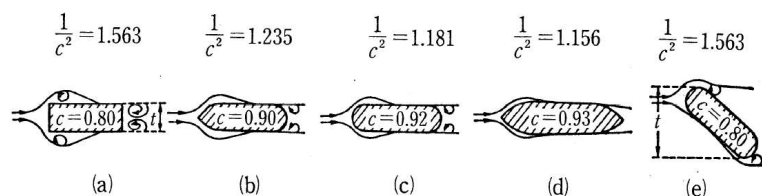
図 3-3 橋脚の形状と C の値 (参考値)
