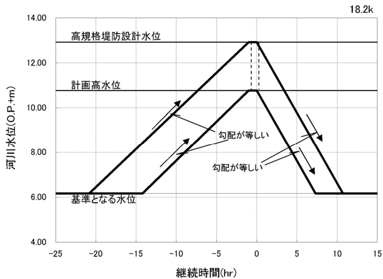
図 5.4.2-2 高規格堤防設計水位に対応した外水波形
