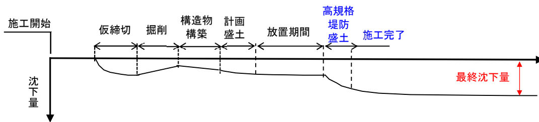
図 5.2.2-8 最終沈下量の考え方
