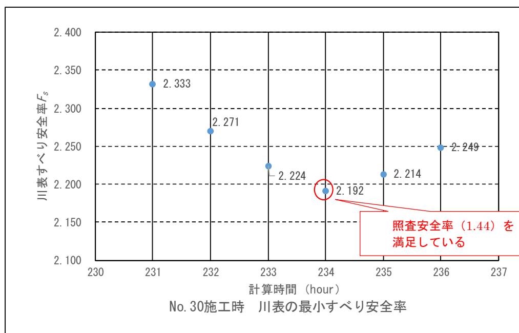
図 6.3.3-2 川表のすべり安全率の経時変化 (No. 30)
