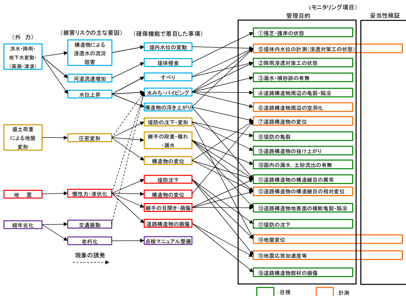
図 7.1.3-1 モニタリング項目の整理
