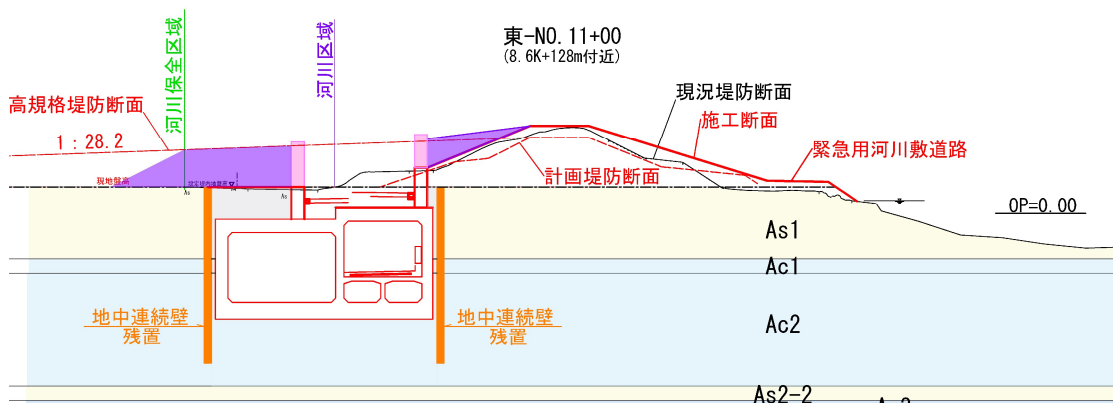
図 5.4.2-11 耐越水性検討断面 (No. 11 8.6k+128m 付近)
