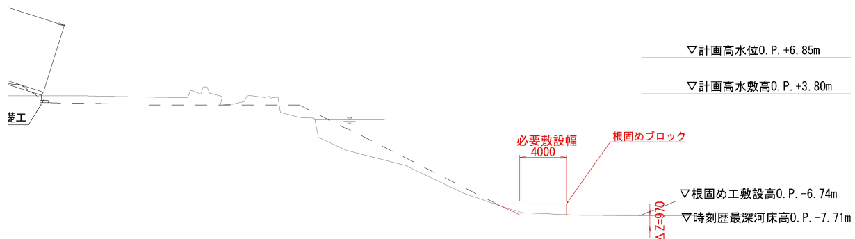
図 6.3.1-9 根固め工敷設幅の検証 (河川距離標：8.4k+197m 道路測点：No.6)
