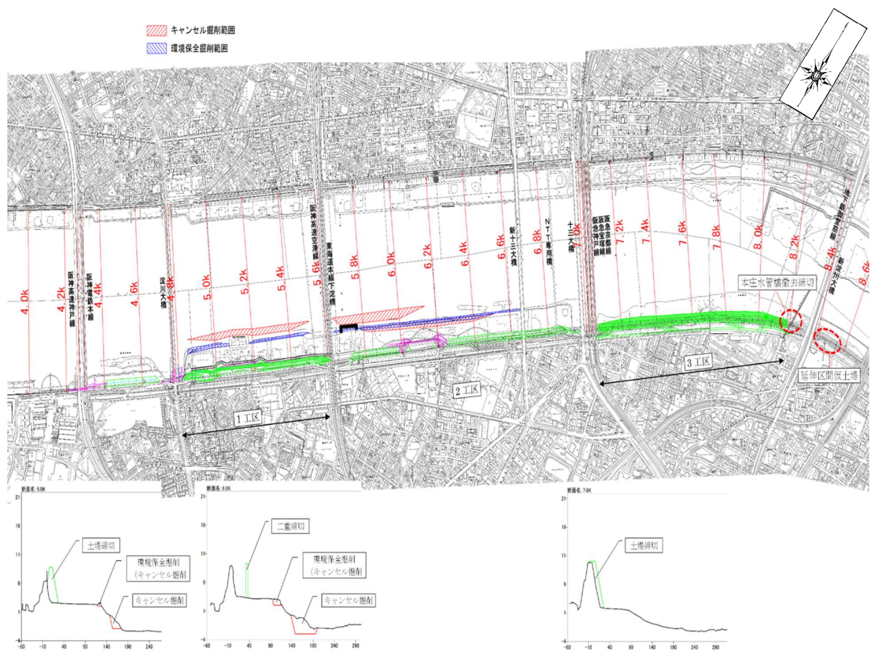
図 6.3.2-2 2 期の仮締切堤とキャンセル掘削の概要
