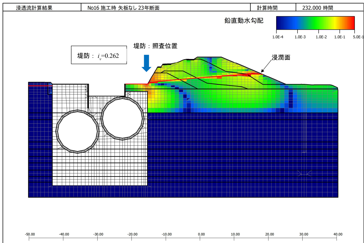
図 6.3.3-6 堤体内水位ピーク時の局所動水勾配コンター (No. 16 施工時)
