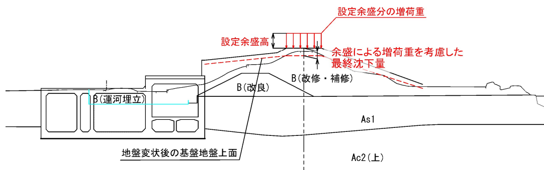
図 5.2.2-9 圧密沈下に伴う堤防高の確保の照査方法
