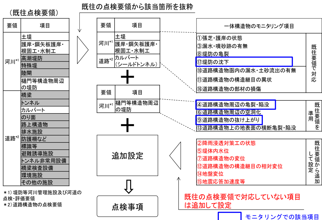
図 7.3.5-1 管理モニタリングにおける不同沈下の該当項目（表 7.3.1-2 再掲, 加筆）
