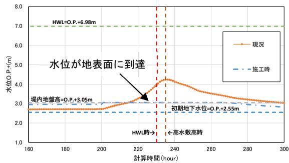
土留め壁前面（河川側）の水位の経時変化
