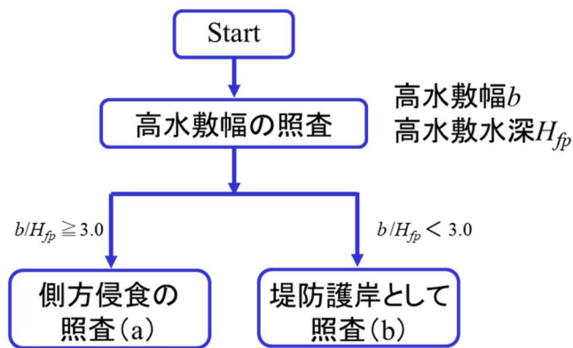
図 6.3.1-7 高水敷幅の照査
