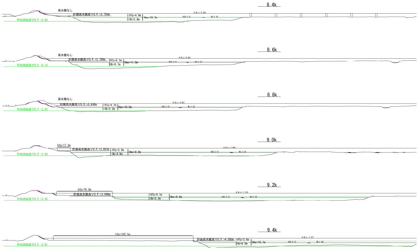
図 6.3.1-2 施工時の河道横断図
