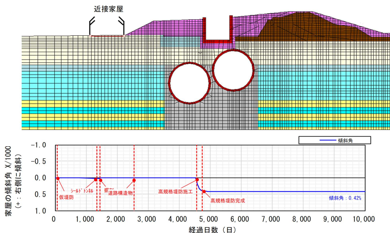
図 5.2.2-11 近接家屋位置における傾斜角の経時変化
