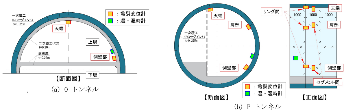
図 7.3.4-5 シールドトンネル内のセグメント目地部の計測機設置事例
