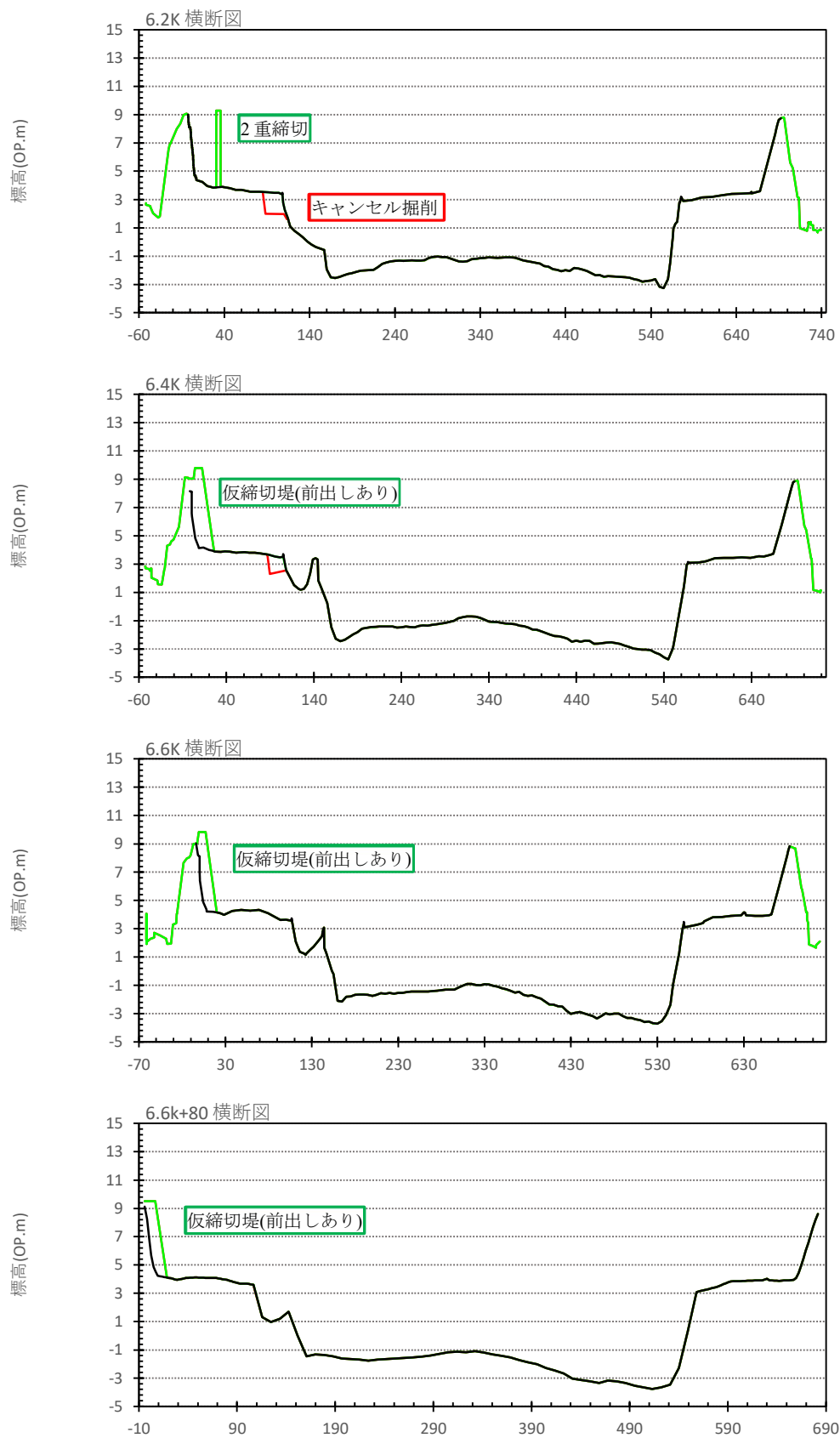
図 6.3.2-3 (5) 不等流計算横断(3.8k~9.2k)
