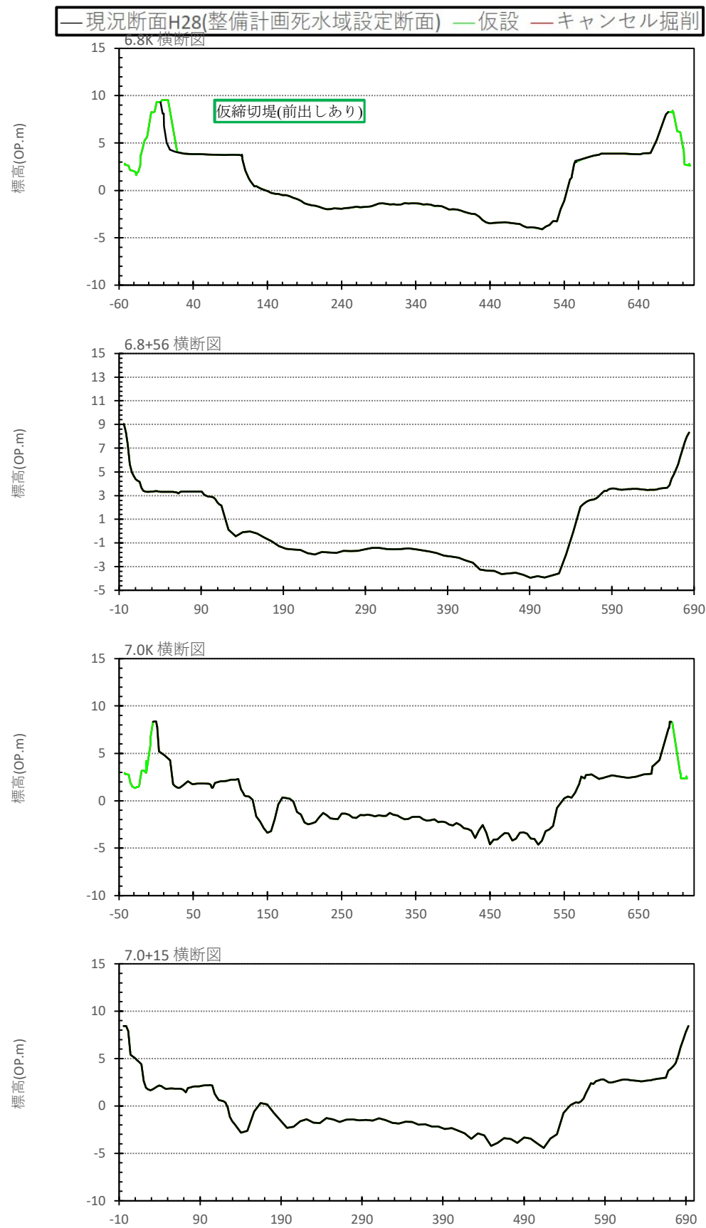
図 6.3.2-3 (6) 不等流計算横断(3.8k~9.2k)
