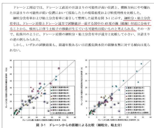
ドレーン工周辺の堤体土の粒度組成変化について (「河川堤防の浸透対策工の長期安全性に係る開削調査」より抜粋)
