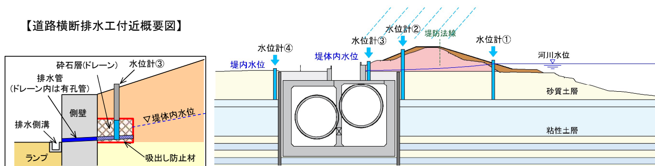
図 7.2.1-1 解析の妥当性検証に用いる水位計測箇所（開削ボックス区間）
