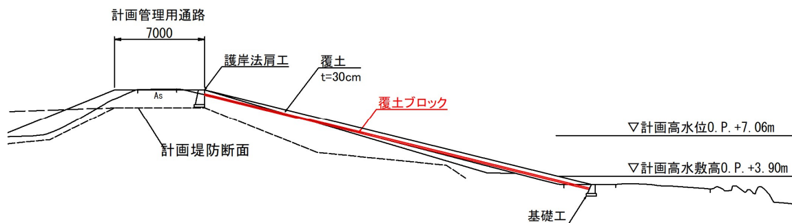
図 5. 4. 2-6 高水護岸部の標準断面図(河川距離標 : 9.0k+4 道路測点 No.24)
