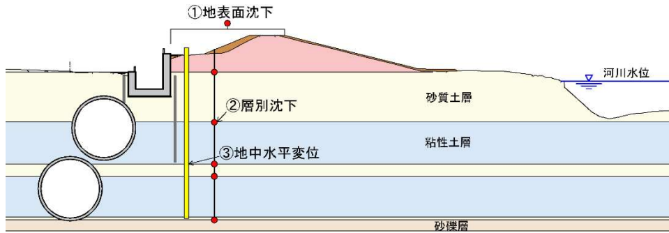
図 7.2.2-2 解析の妥当性検証に用いる地盤変位計測箇所（シールドトンネル区間）
