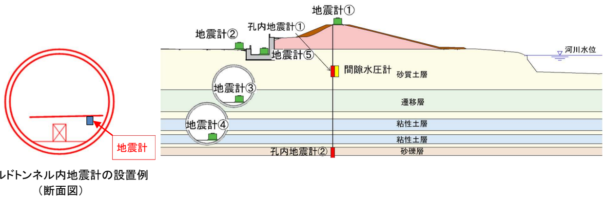
図 7.2.3-2 地震計と間隙水圧計の設置例（シールドトンネル区間）
