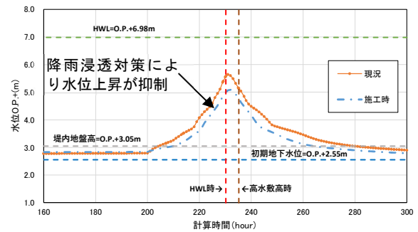
堤防天端中央の水位の経時変化
