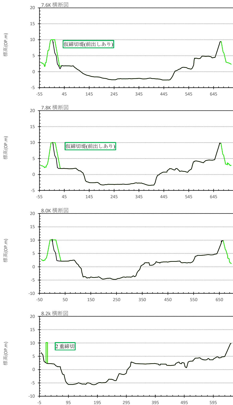
図 6.3.2-3 (8) 不等流計算横断(3.8k~9.2k)
