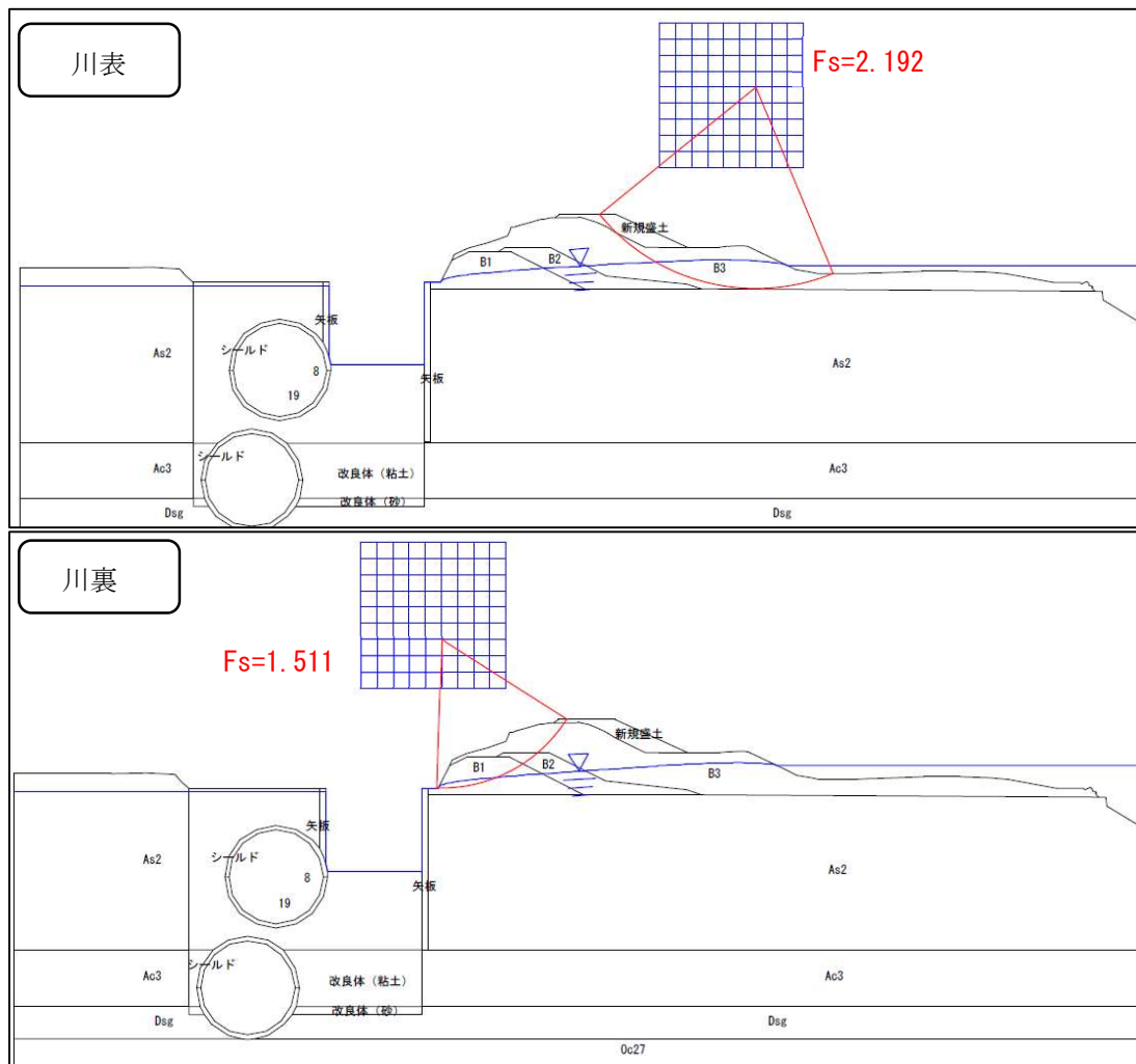
図 6.3.3-3 すべり安全率結果 (No. 30) (上：川表，下：川裏)
