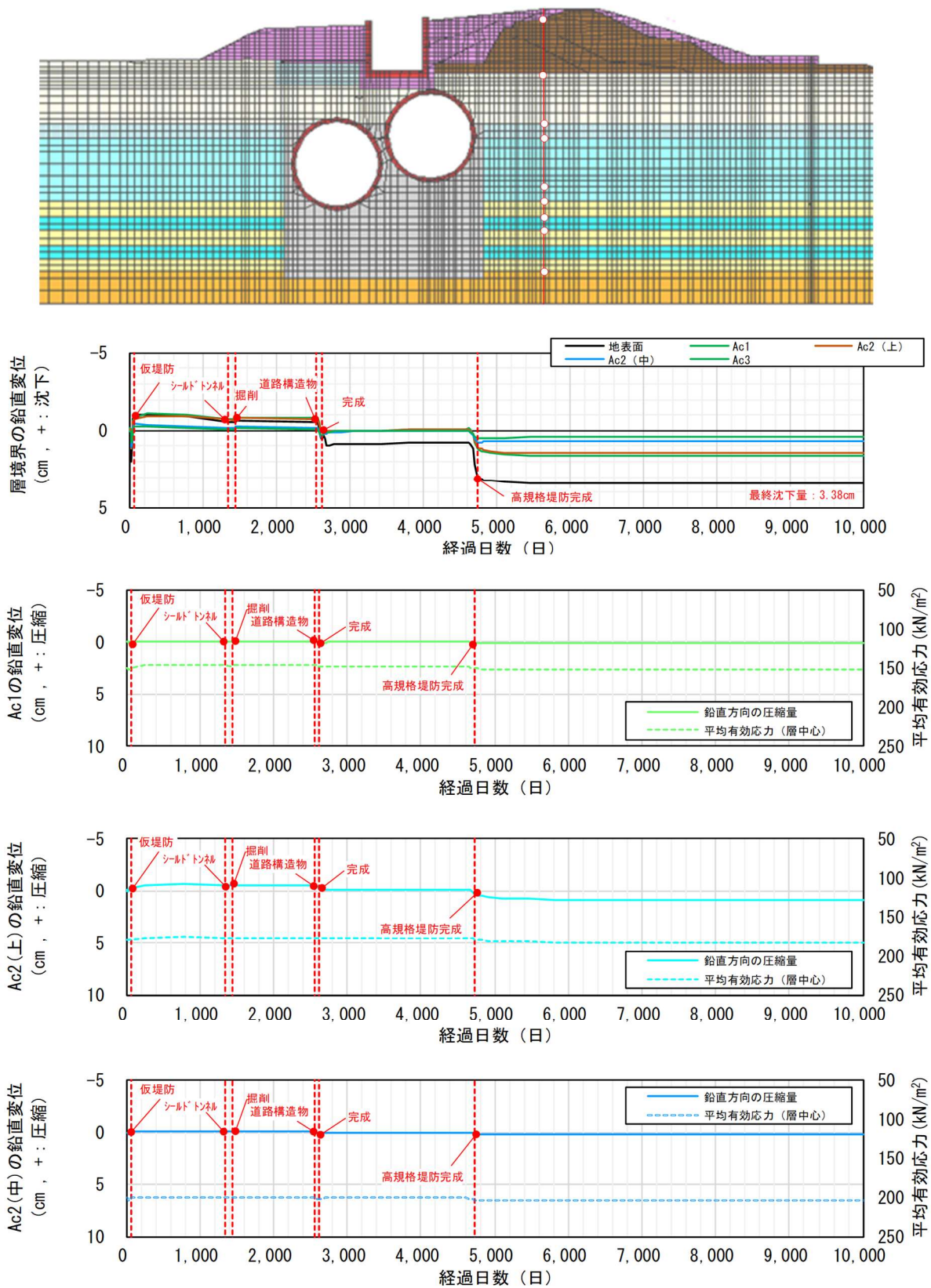
図 5.2.2-10 堤防天端位置における地盤変状挙動，応力状態の経時変化
