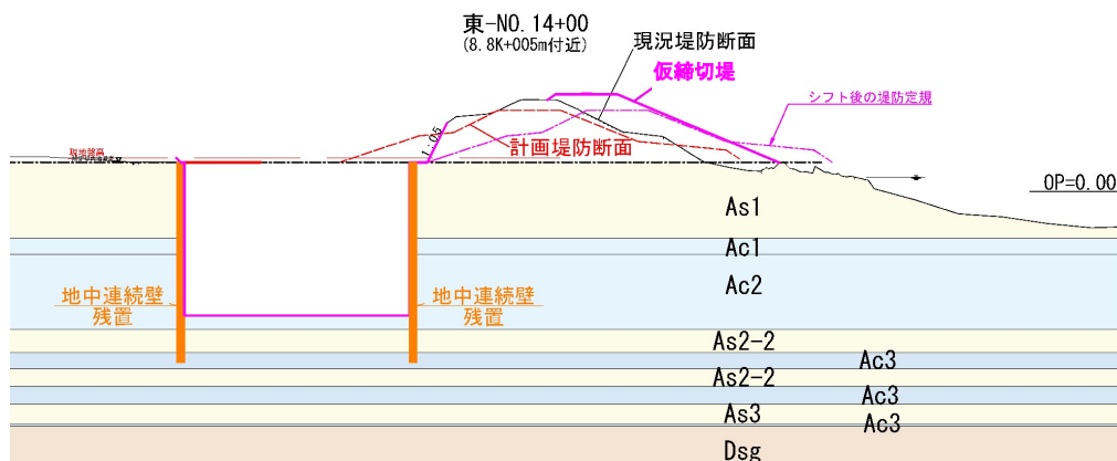
図 6.2-1 延伸部区間における土堤仮締切状況
