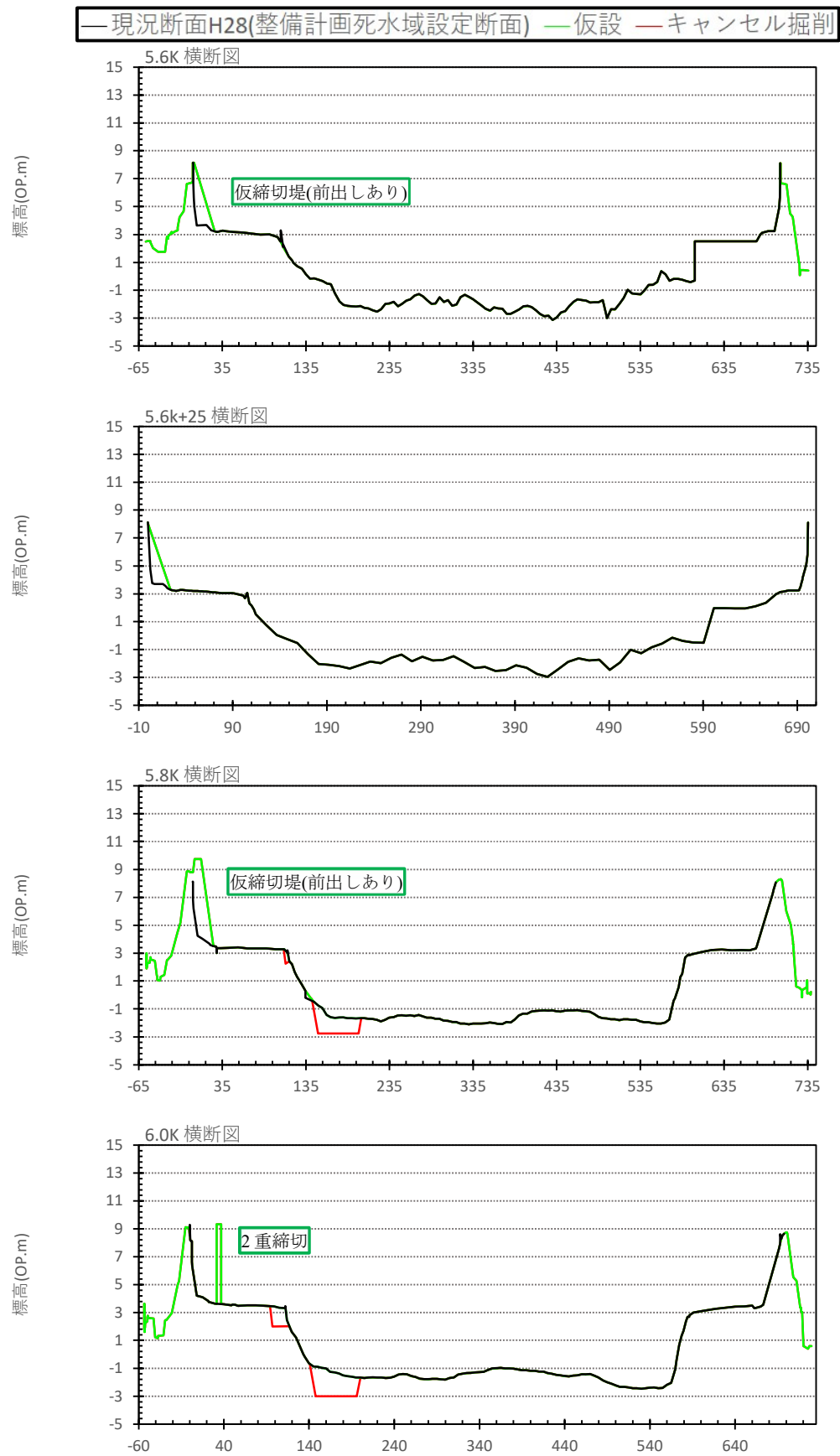
図 6.3.2-3 (4) 不等流計算横断(3.8k~9.2k)
