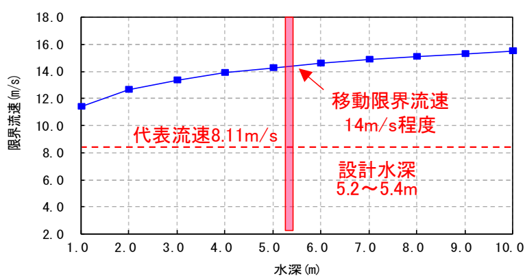
図 5.4.2-8 水深と限界流速の関係（堤防護岸における大型連節ブロック）
