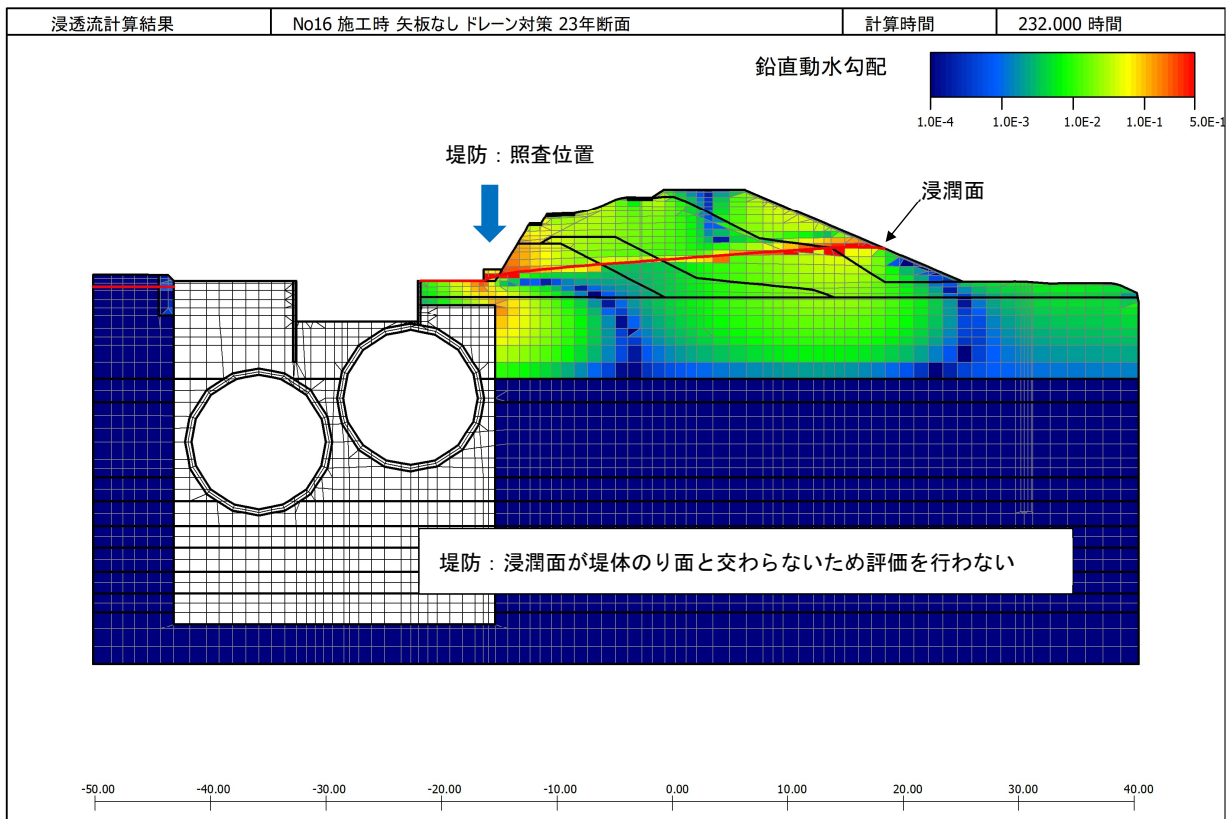
図 6.3.3-7 堤体内水位ピーク時の局所動水勾配コンター (No. 16 施工時 ドレーン工)
