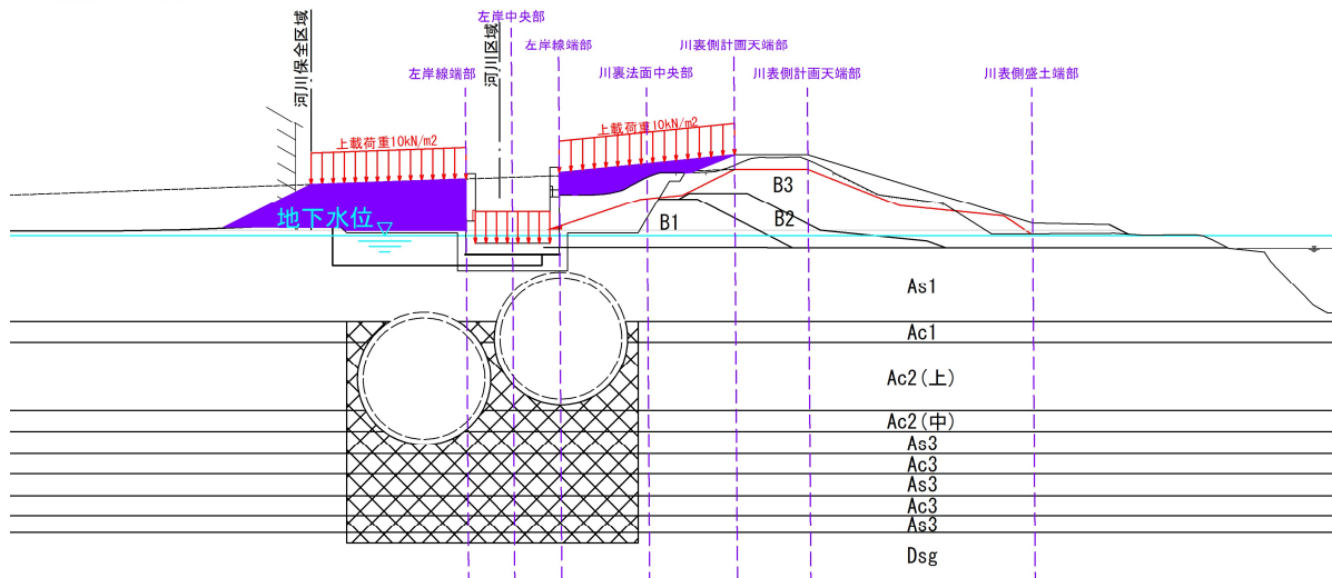
図 5.2.2-6 解析モデル図 (No. 16)
