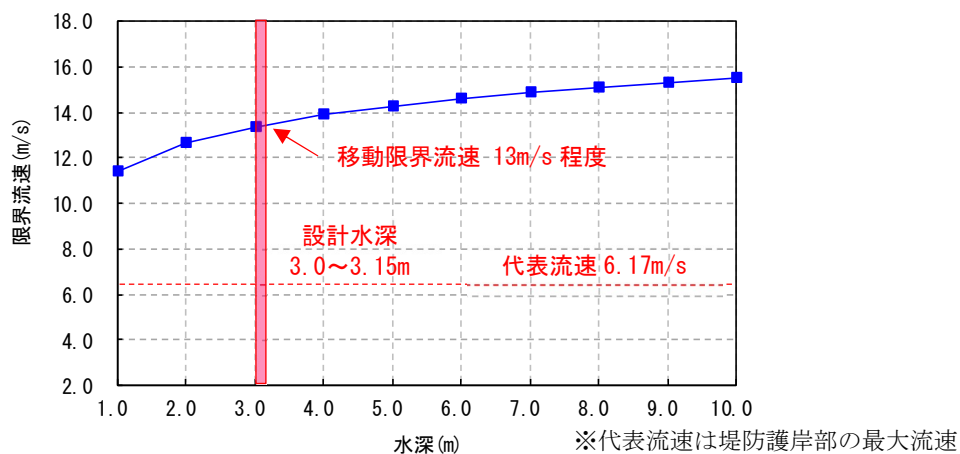
図 6.3.1-3 水深と限界流速の関係（堤防護岸における大型連節ブロック）
