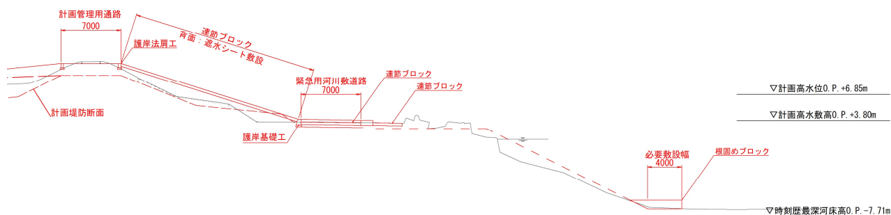
図 5. 4. 2-5 堤防護岸部の標準断面図(河川距離標 : 8.4k+197m 道路測点 : No. 6)
