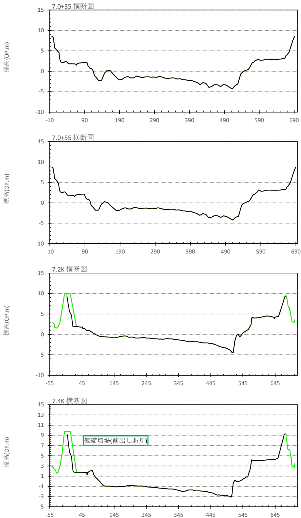
図 6.3.2-3 (7) 不等流計算横断(3.8k~9.2k)
