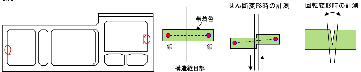
図 7.3.4-4 道路構造物上部の横断方向の段差に関するモニタリング項目
