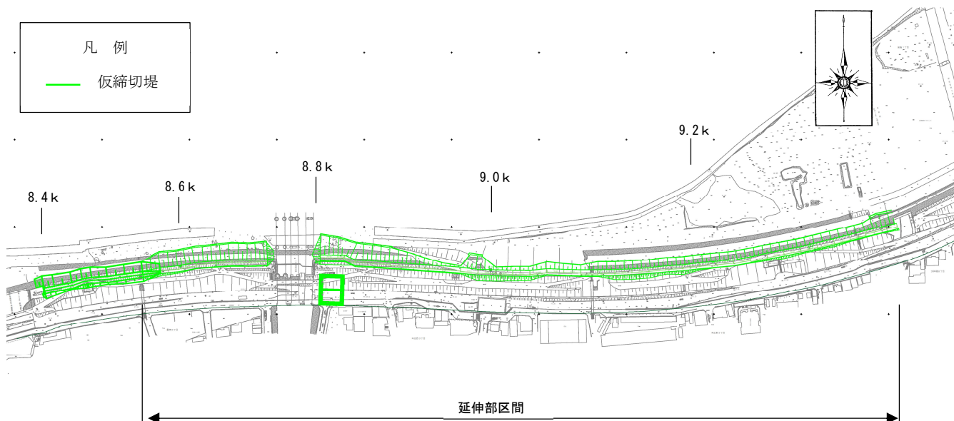
仮締切堤平面図
