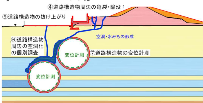
図 7.3.4-3 堤防と道路構造物の境界に関するモニタリング項目
