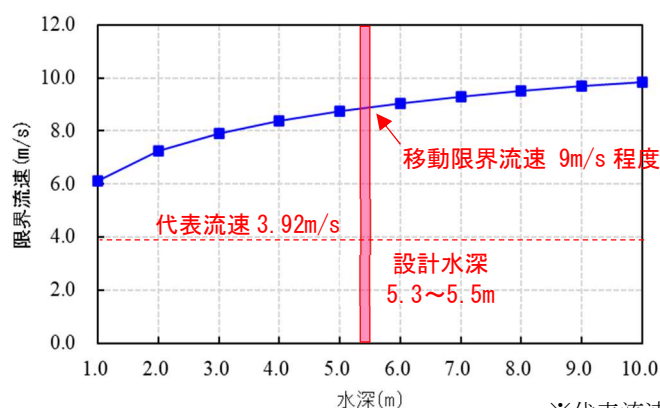
図 5.4.2-9 水深と限界流速の関係（高水護岸における覆土ブロック）
