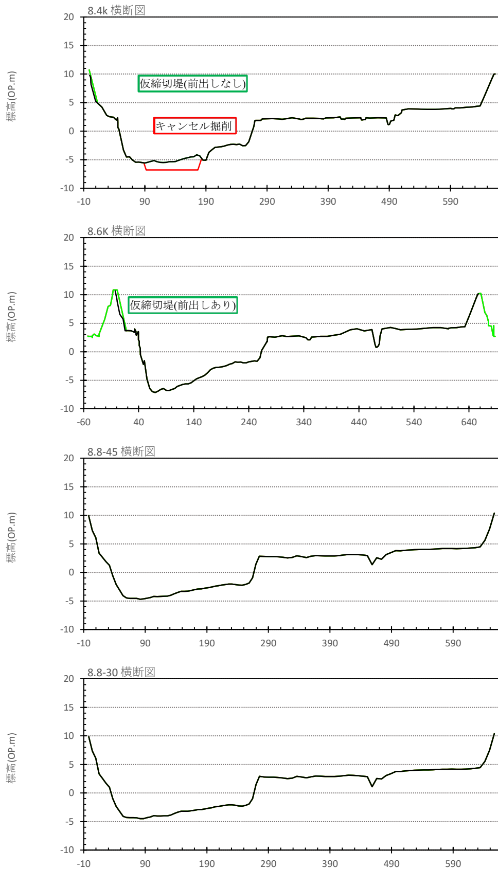
図 6.3.2-3 (9) 不等流計算横断(3.8k~9.2k)
