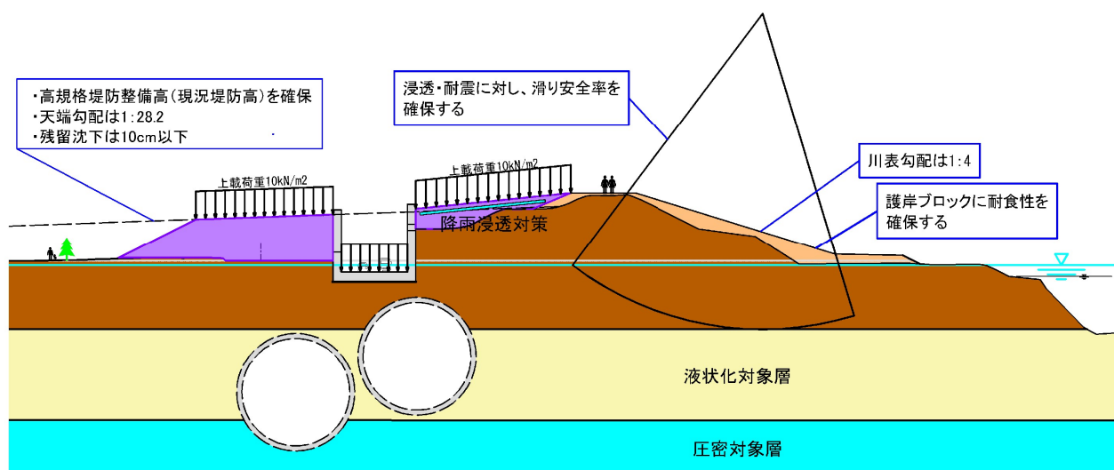
図 5.4.2-1 高規格堤防のイメージ
