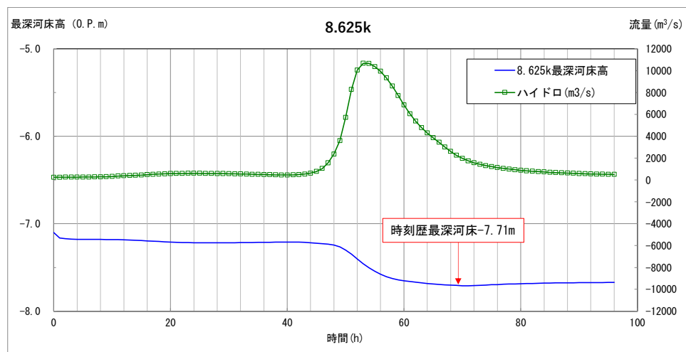
図 6.3.1-8 河床変動解析に基づく最深河床高縦断面図
