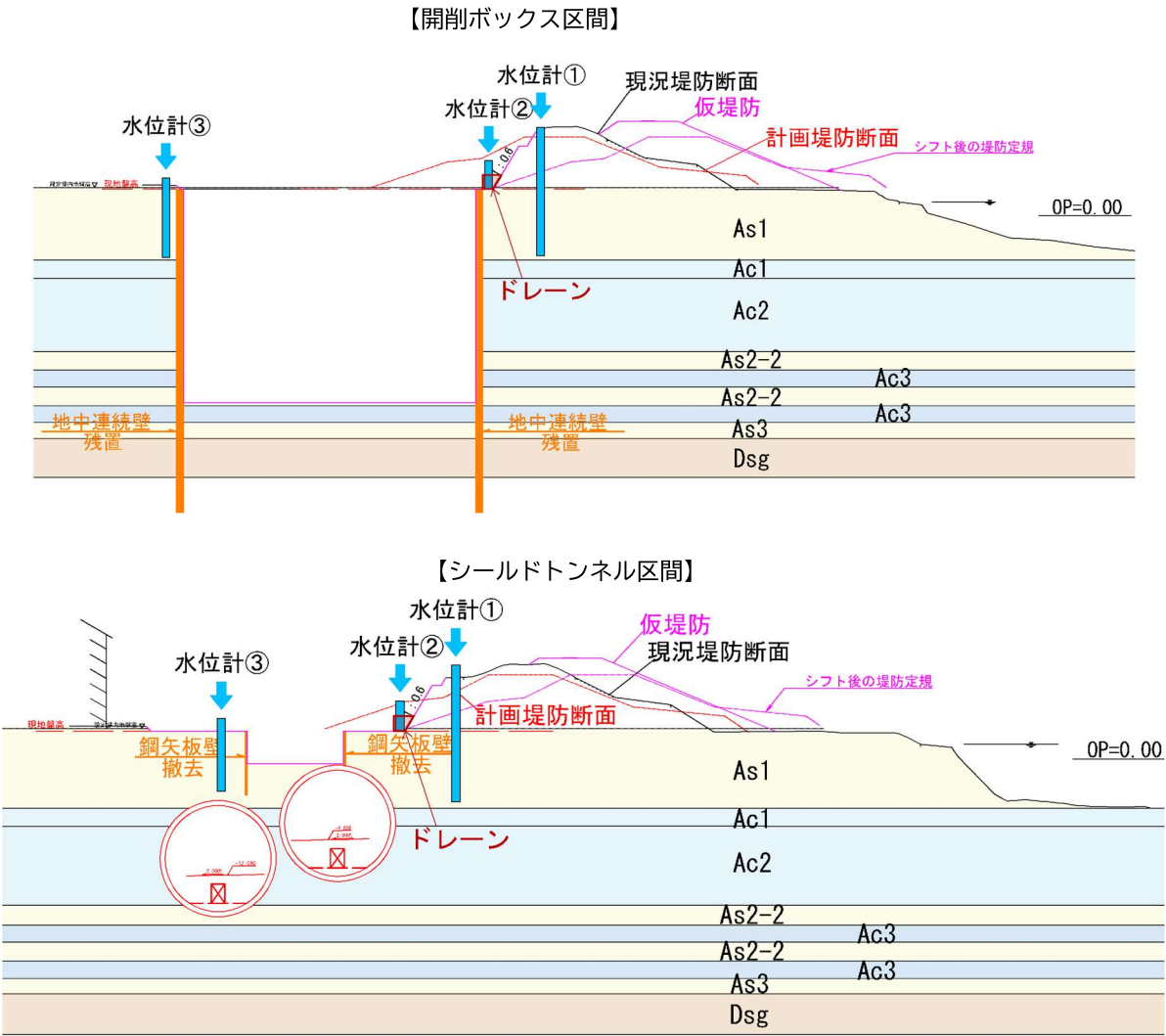
図 6.4.3-1 施工時の水位計測例
