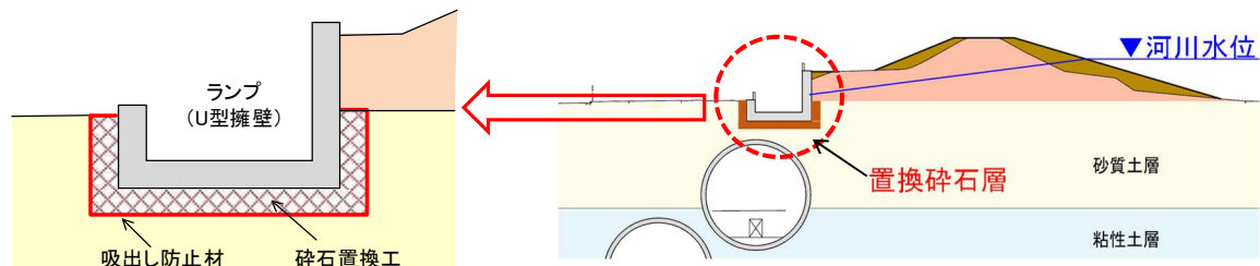
図 7.3.5-5 砕石置換工概要図
