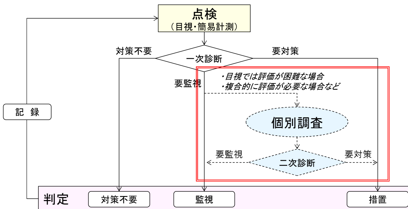
図 7.3.4-1 点検結果の評価の流れ
