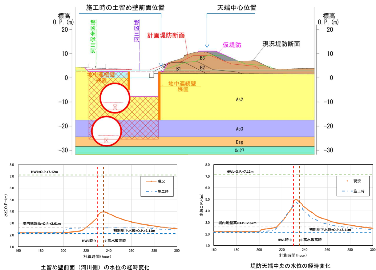
図 6.3.3-1 堤体内水位の経時変化の比較 (No. 30)
