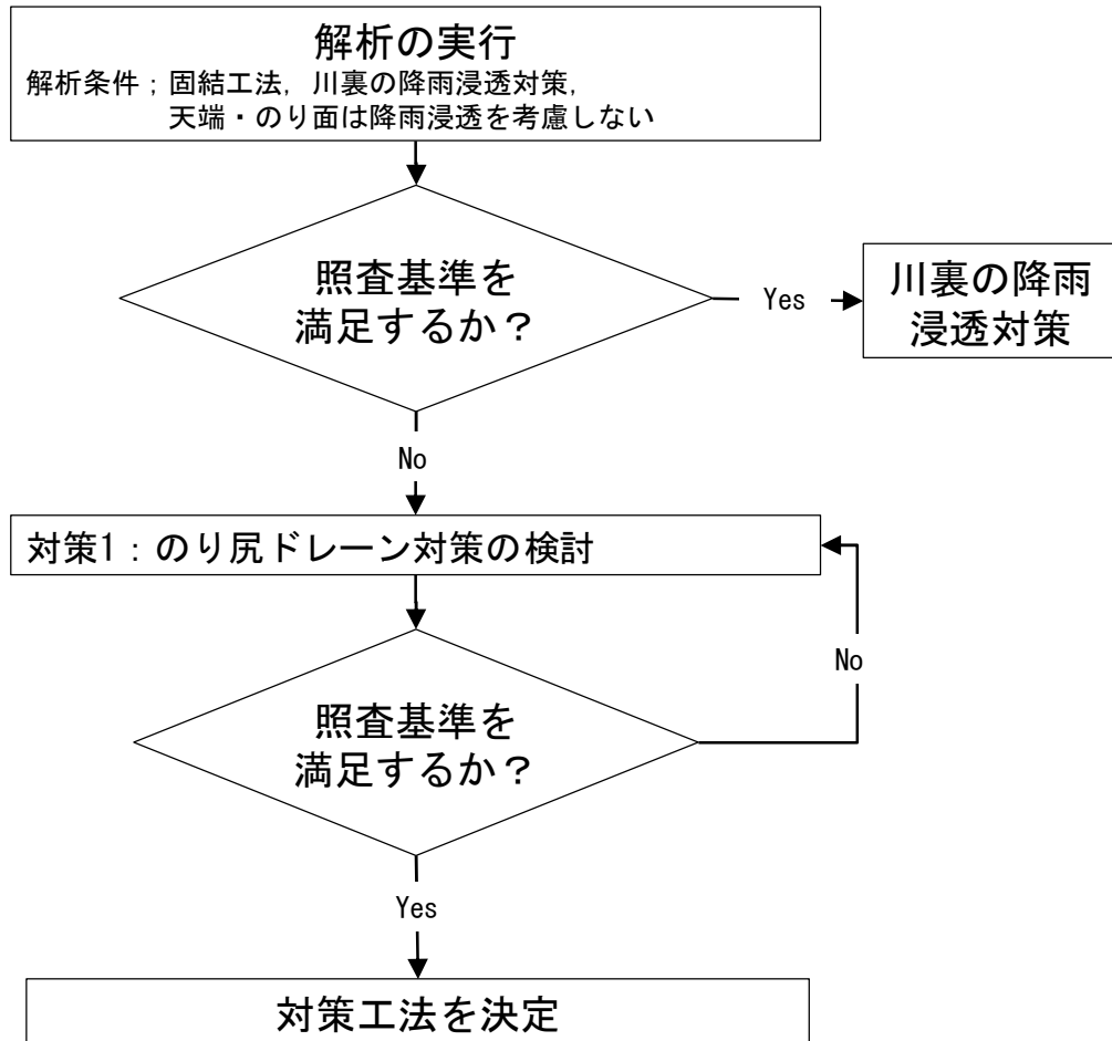
図 6.3.3-5 浸透対策工（局所動水勾配対策）の検討フロー
