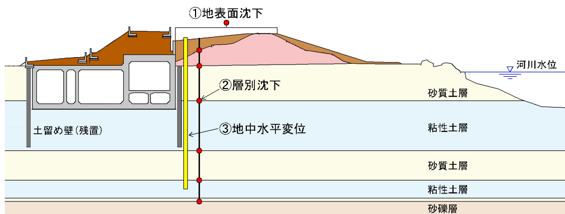
図 7.2.2-1 解析の妥当性検証に用いる地盤変位計測箇所（開削ボックス区間）
