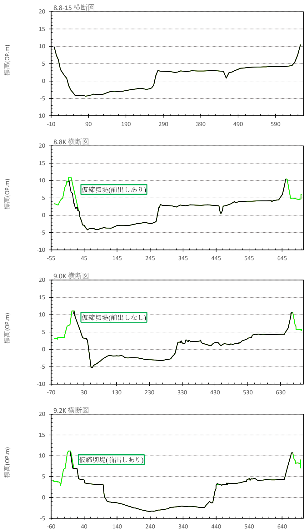
図 6.3.2-3 (10) 不等流計算横断(3.8k~9.2k)
