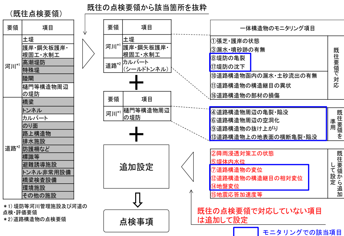
図 7.3.5-3 管理モニタリングにおけるゆるみ・空洞・水みち等の該当項目 (図 7.3.1-2 再掲, 加筆)
