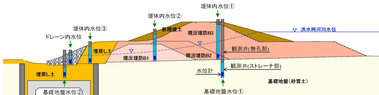
図 7.3.5-7 のり尻ドレーン設置区間の水位観測孔配置例
