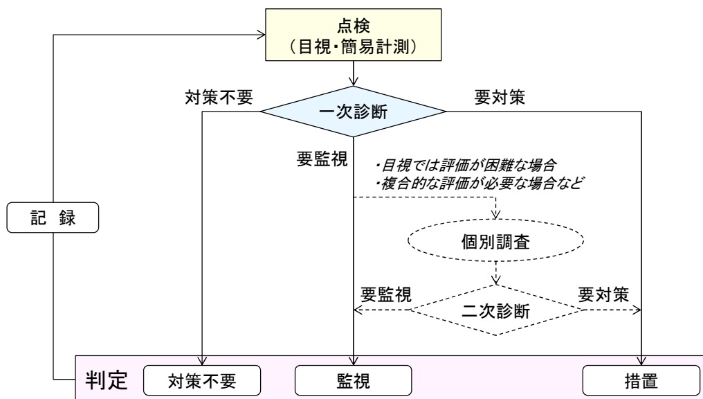
図 7.3.2-1 点検結果の評価の流れ
